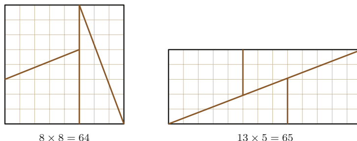
Рис. 0.6. Квадрат 8 \times 8 и прямоугольник 13 \times 5 , сложенный из тех же четырёх частей. Ни одна не потерялась и ни одна не добавилась.
